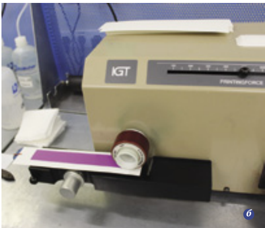
Рис. 3. Фрагменты проводимых в лаборатории качества типографии «Промис» работ: а — взвешивание требуемого количества краски; б — получение тестовой полосы на пробпечатном офсетном станке; в — измерение цветовых характеристик тестовой полосы спектрофотометром; г — визуальный тест правильности воспроизведения цветов на печатном оттиске
